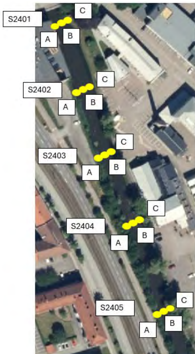
Figur 3 Provtagningspunkter sediment.
