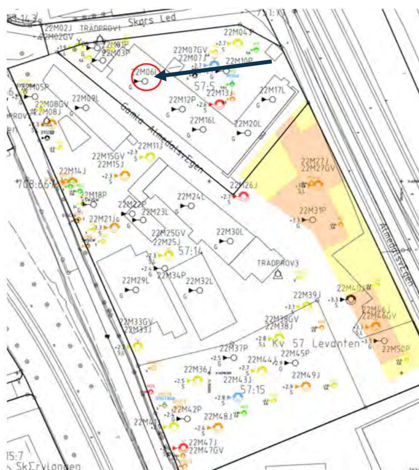
Figur 5. Inomhusluftprovtagningen
